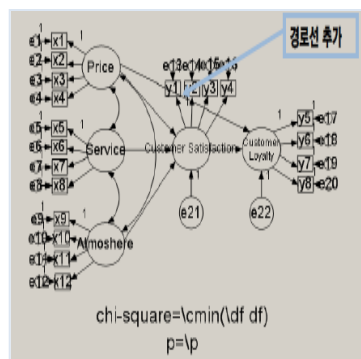
[수정모형 고려]
