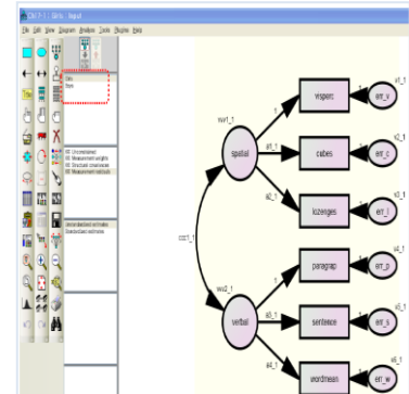
[다중집단분석]
