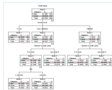
[CHAID 방법]
